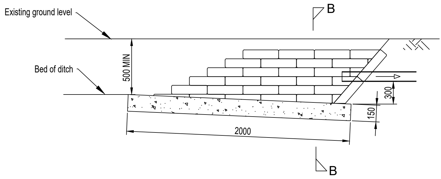
LONGITUDINAL PROFILE
